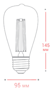
Чертеж размеров
